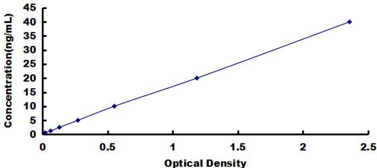
人脂蛋白脂酶(LIPD)检测试剂盒标准曲线
