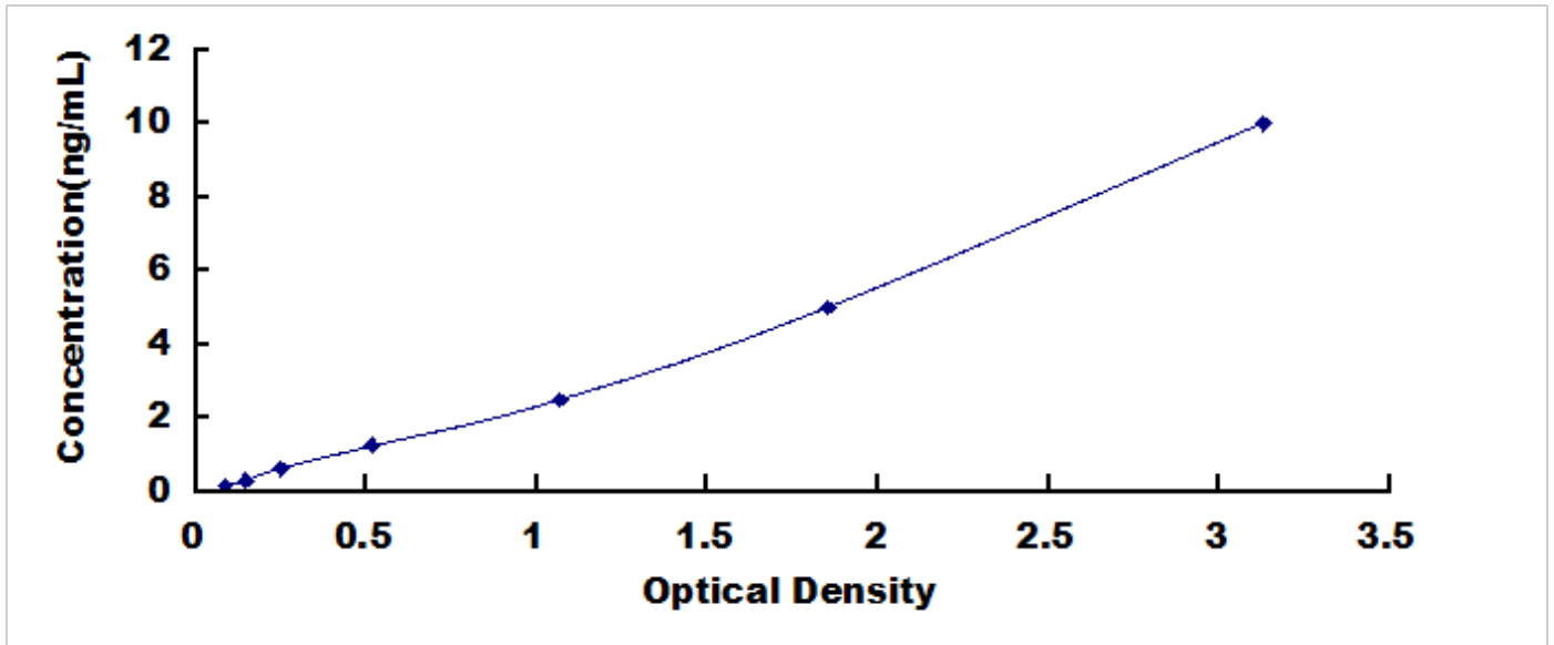
人肝表达抗菌肽 2 (LEAP2) 检测试剂盒标准曲线
