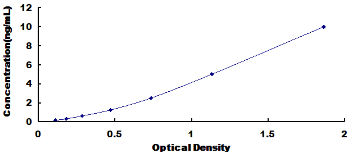
人肝 X 受体 \alpha (LXR \alpha ) 检测试剂盒标准曲线
