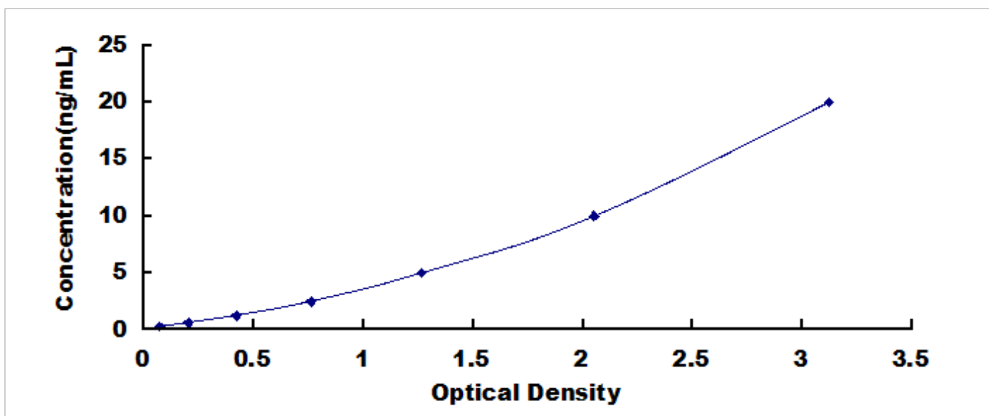
人基膜聚糖 (LUM) 检测试剂盒标准曲线
