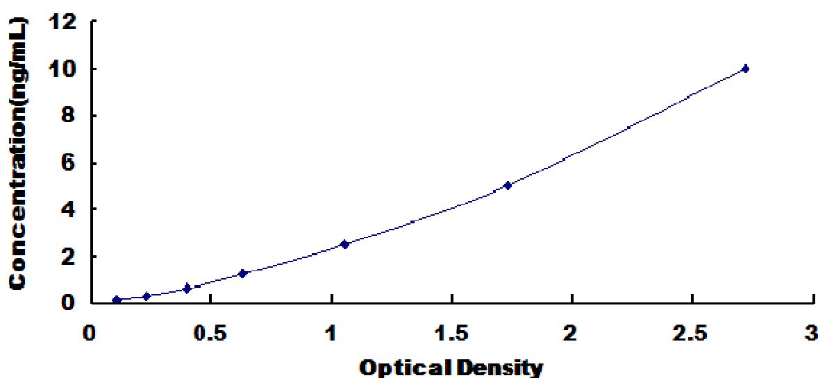
小鼠溶菌酶(LZM)检测试剂盒标准曲线
