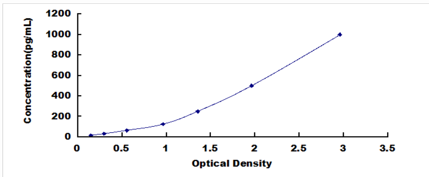
人赖氨酰氧化酶(LOX)检测试剂盒标准曲线
