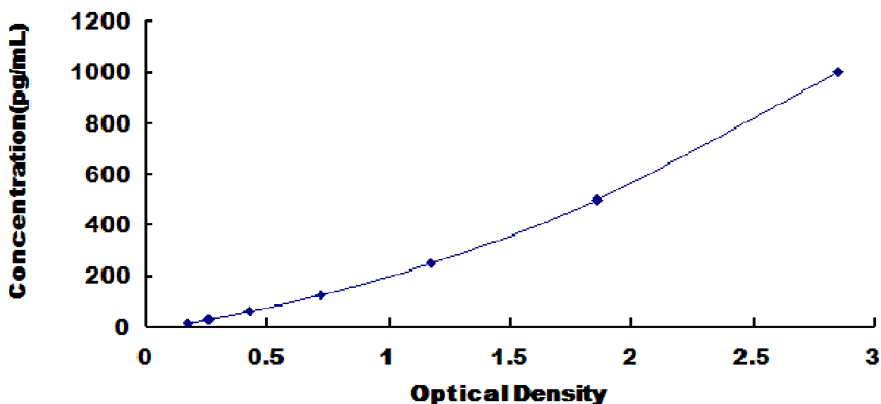
人巨噬细胞炎性蛋白 1 \alpha (MIP1 \alpha ) 检测试剂盒标准曲线
