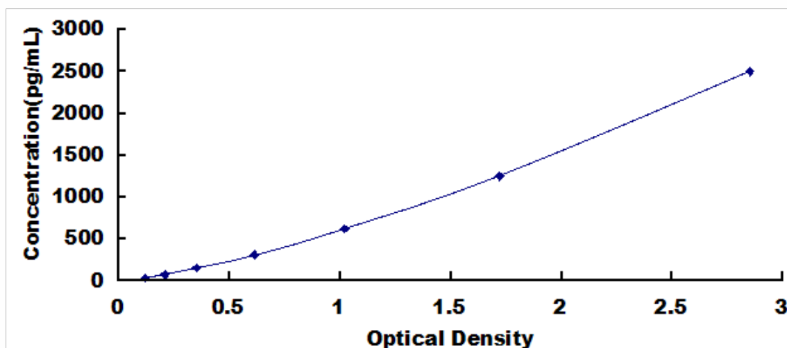
小鼠 II 类主要组织相容性复合体 DR β 1 (MHC DR β 1) 试剂盒标准曲线
