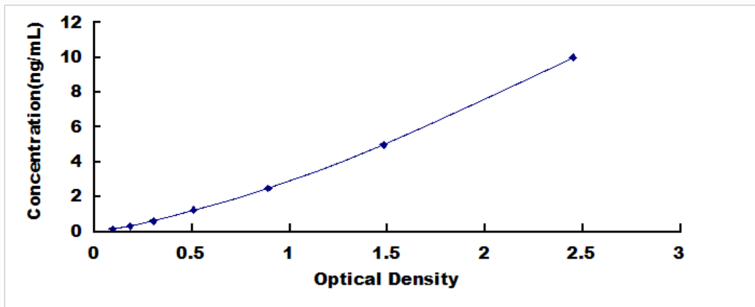
人甘露糖结合蛋白 (MBL) 检测试剂盒标准曲线
