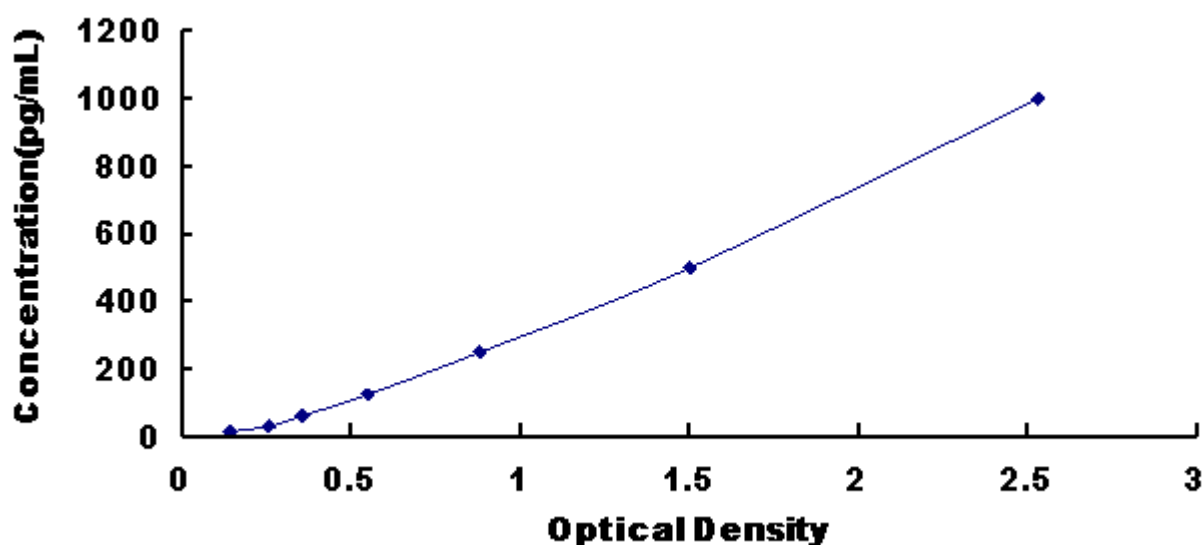
大鼠基质金属蛋白酶 13(MMP13)试剂盒标准曲线
