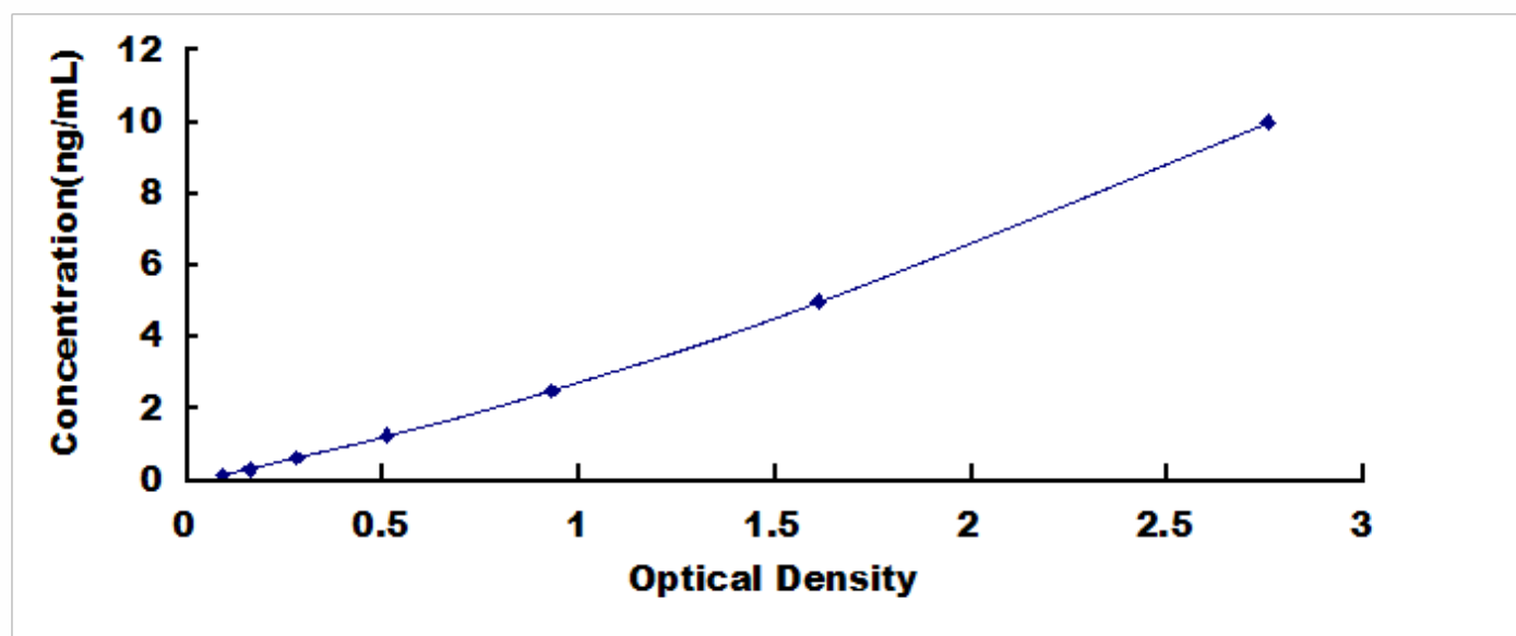
大鼠基质金属蛋白酶 13(MMP13)检测试剂盒标准曲线
