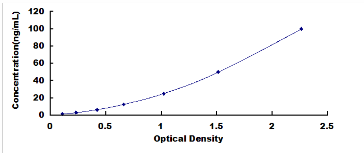
人基质金属蛋白酶 14(MMP14) 检测试剂盒标准曲线
