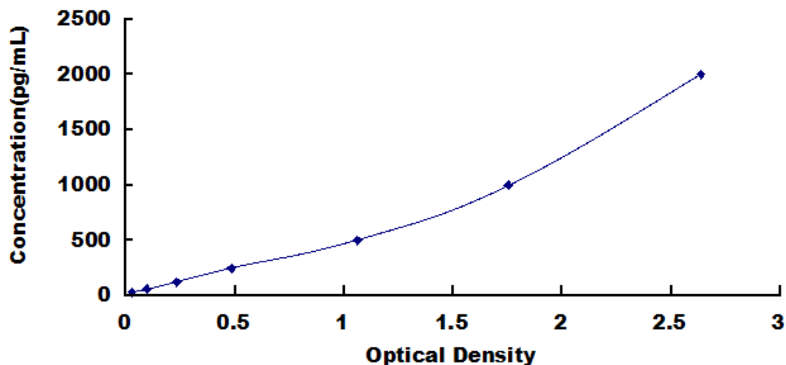
人基质金属蛋白酶 2 (MMP2) 检测试剂盒标准曲线
