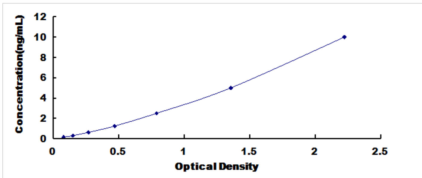
人基质金属蛋白酶 3 (MMP3) 检测试剂盒标准曲线
