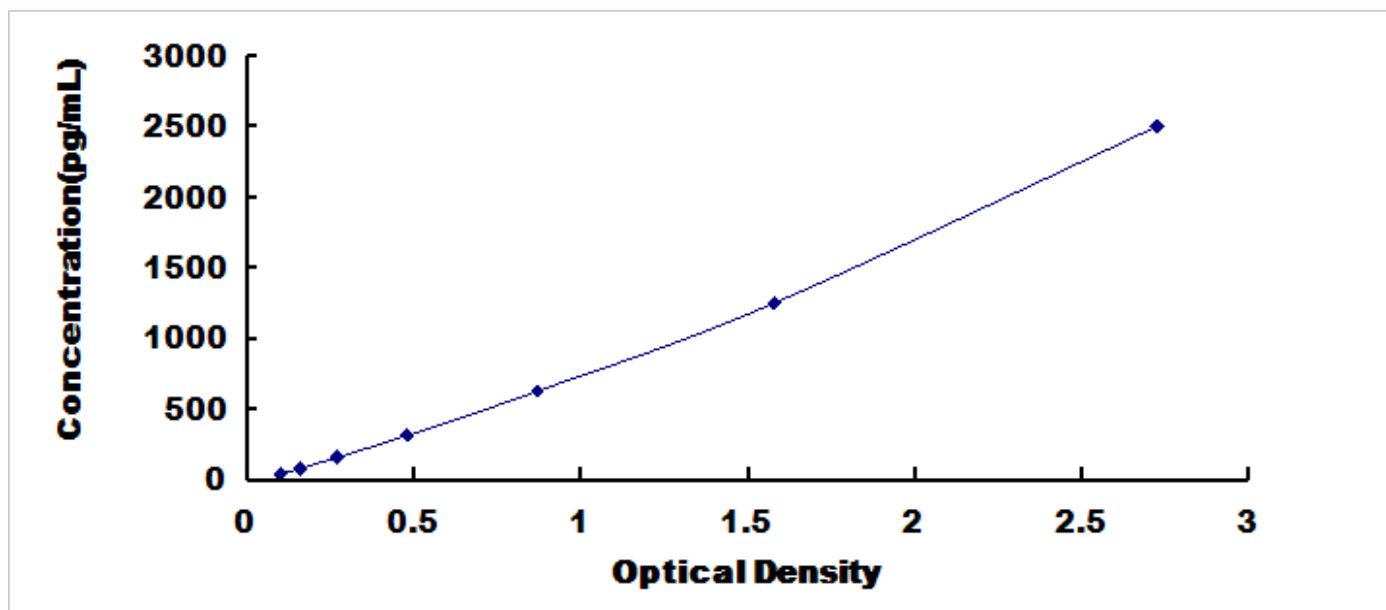
人基质金属蛋白酶 8 (MMP8) 检测试剂盒标准曲线
