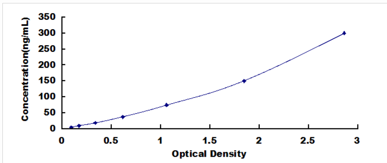
大鼠基质金属蛋白酶 9 (MMP9) 检测试剂盒标准曲线
