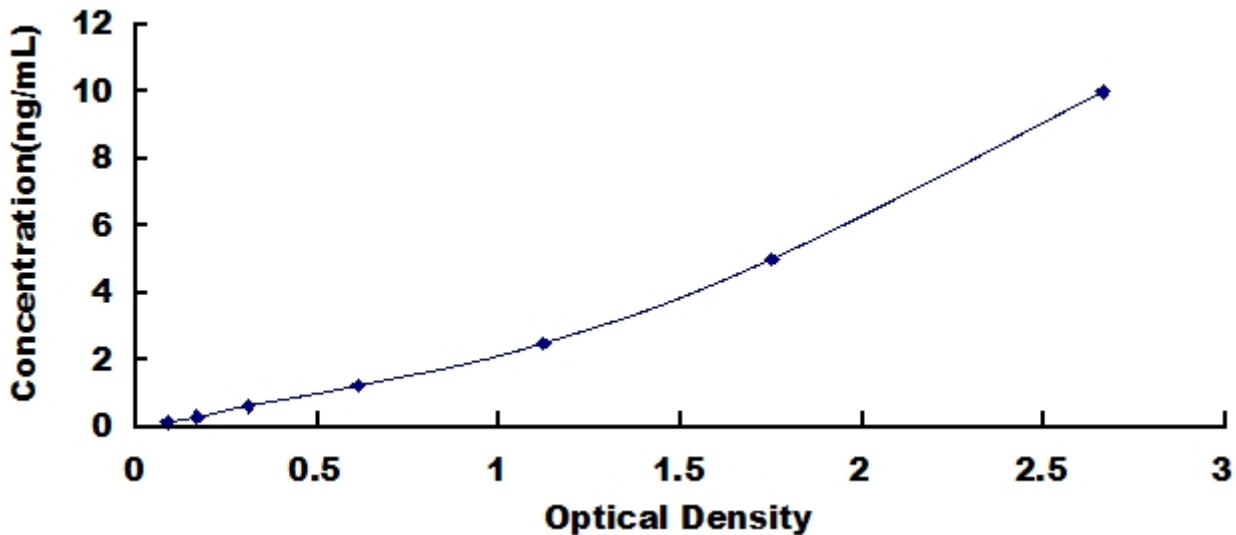
人 Mdm2 p53 结合蛋白同源物 (MDM2) 检测试剂盒标准曲线
