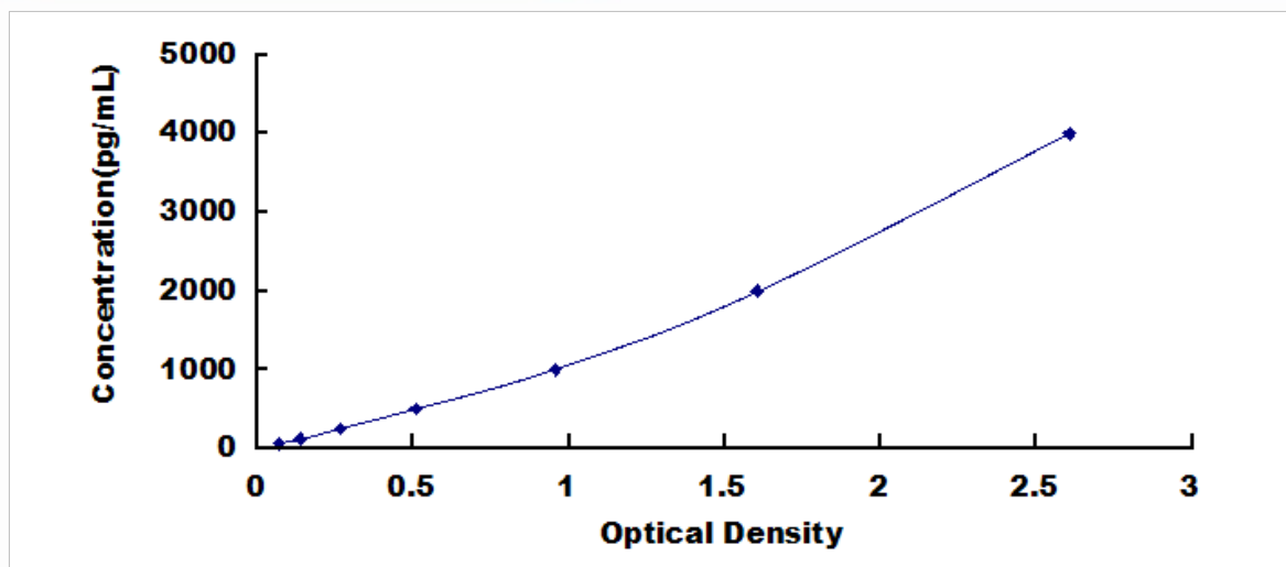
小鼠 MT1 金属硫蛋白 1 (MT1) 检测试剂盒标准曲线
