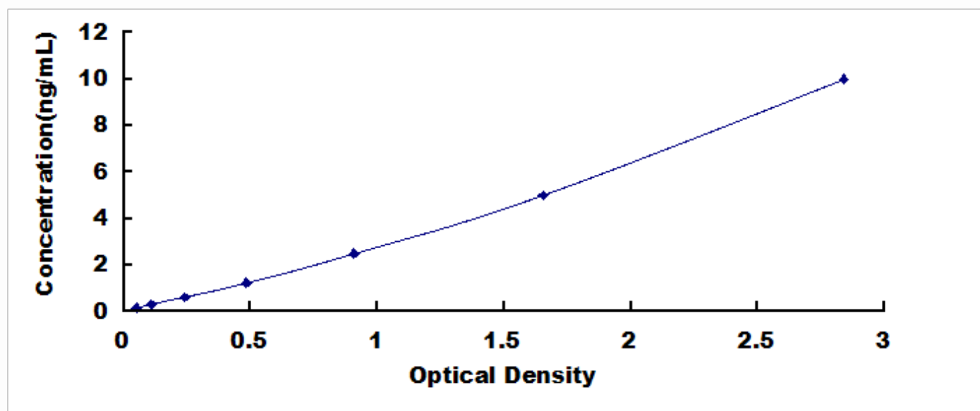
人金属硫蛋白 3(MT3)检测试剂盒标准曲线
