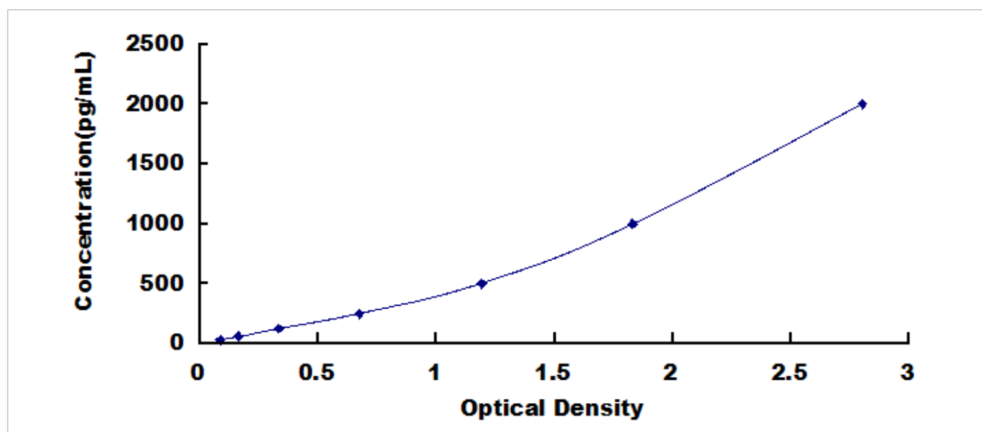
人乳脂球表皮生长因子 8 (MFGE8) 检测试剂盒标准曲线
