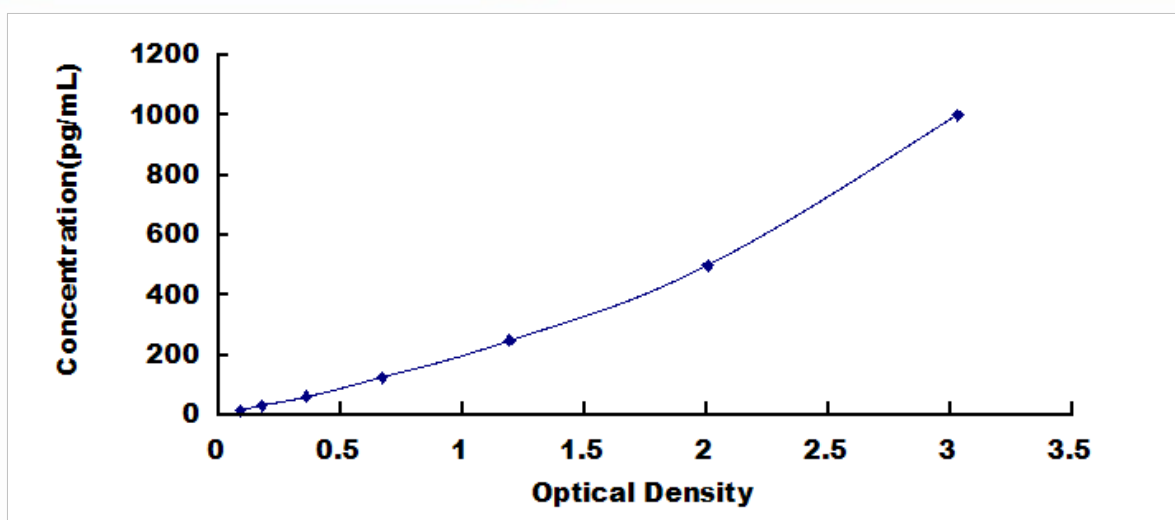
大鼠乳脂球表皮生长因子 8 (MFGE8) 检测试剂盒标准曲线
