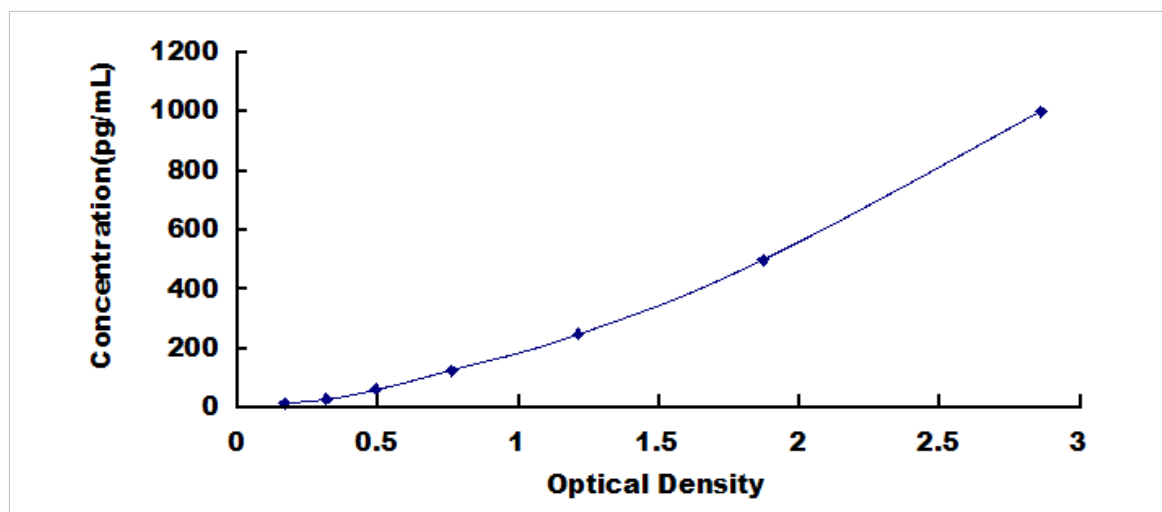
人单核细胞趋化蛋白 1 (MCP1) 检测试剂盒标准曲线
