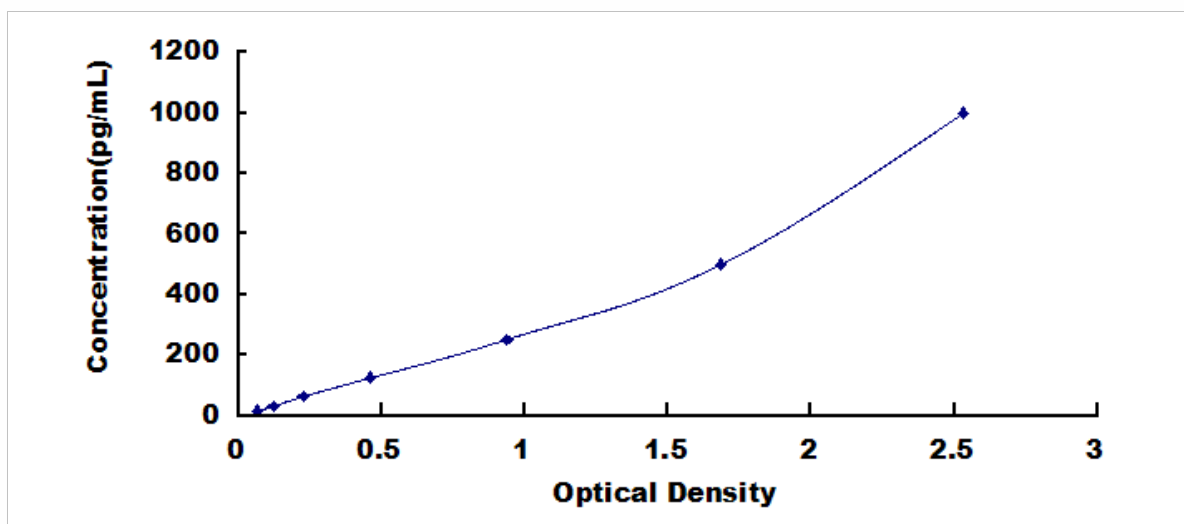
人单核细胞趋化蛋白 2 (MCP2) 检测试剂盒标准曲线
