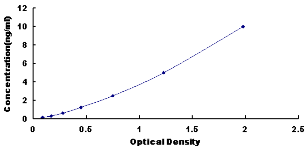
图 1：大鼠 \gamma 干扰素诱导单核因子(MI \gamma )试剂盒标准曲线
