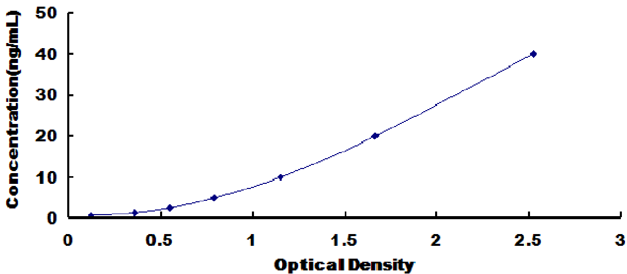
人粘蛋白 5B(MUC5B) 检测试剂盒标准曲线
