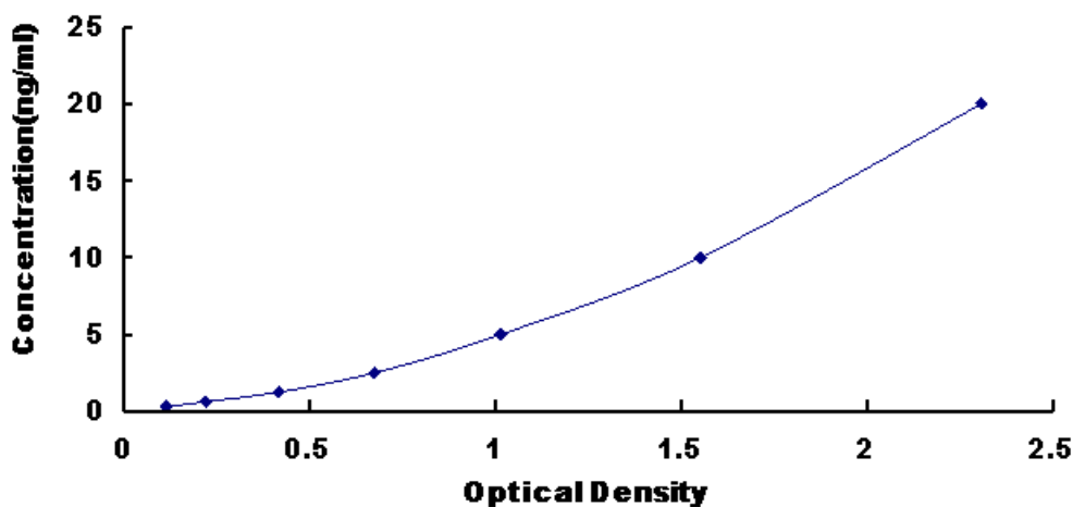
图 1: 小鼠粘蛋白 5B(MUC5B)试剂盒标准曲线
