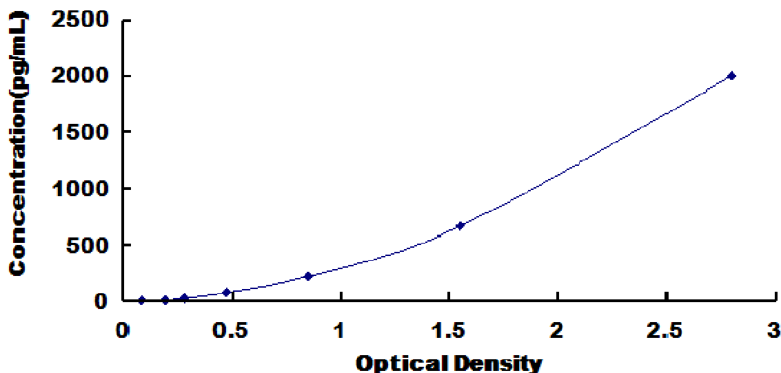
人多聚蛋白 1 (MMRN1) 检测试剂盒标准曲线
