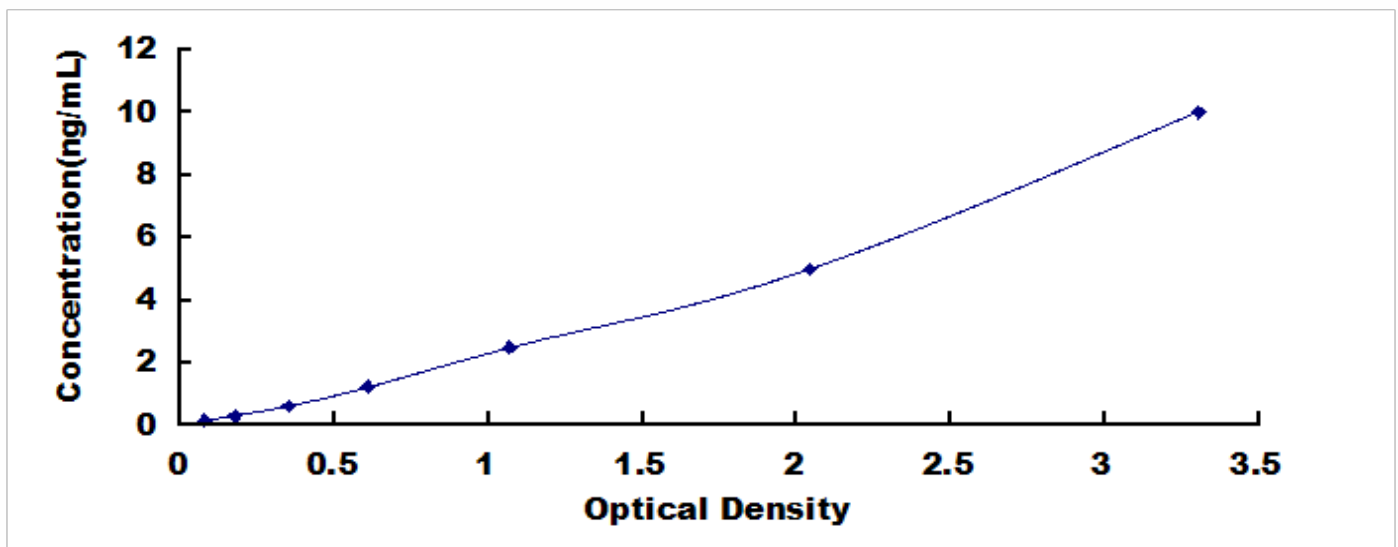
人髓鞘碱性蛋白(MBP)检测试剂盒标准曲线
