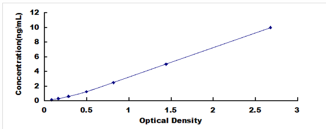
大鼠髓鞘碱性蛋白(MBP)检测试剂盒标准曲线
