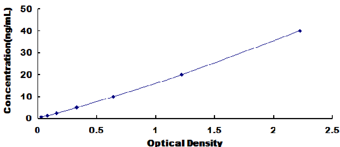
大鼠 N-乙酰转移酶 2 (NAT2) 检测试剂盒标准曲线
