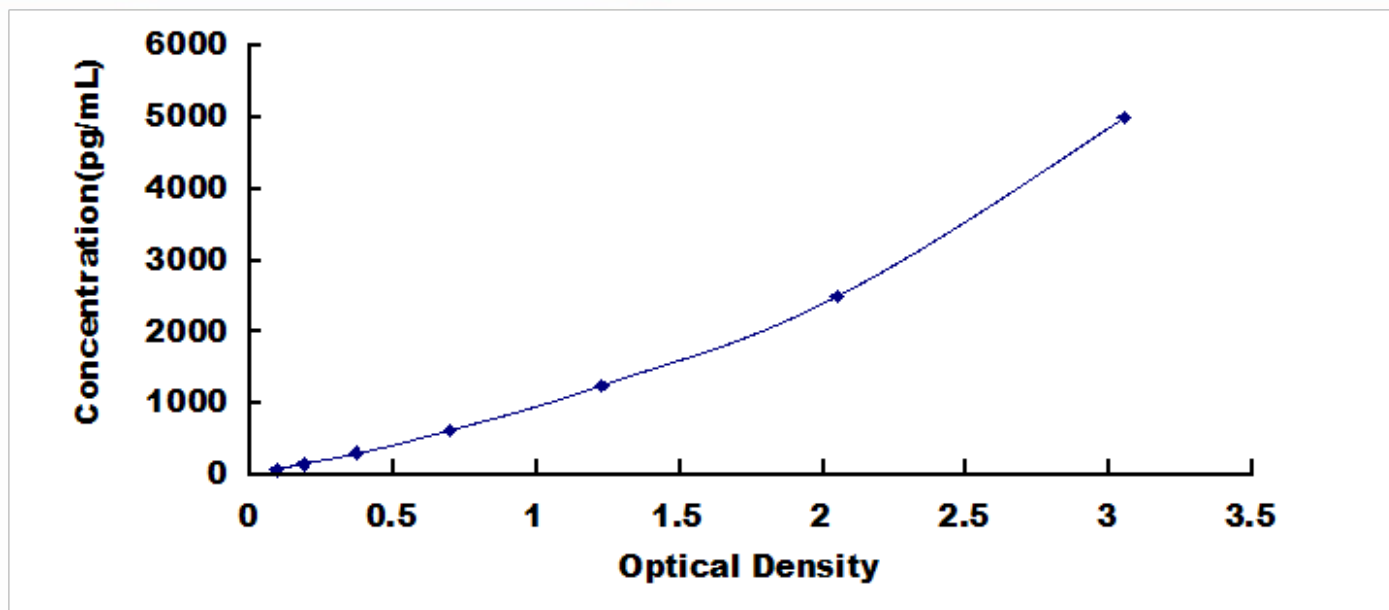
小鼠氨基端前心钠肽 (NT-ProANP) 检测试剂盒标准曲线
