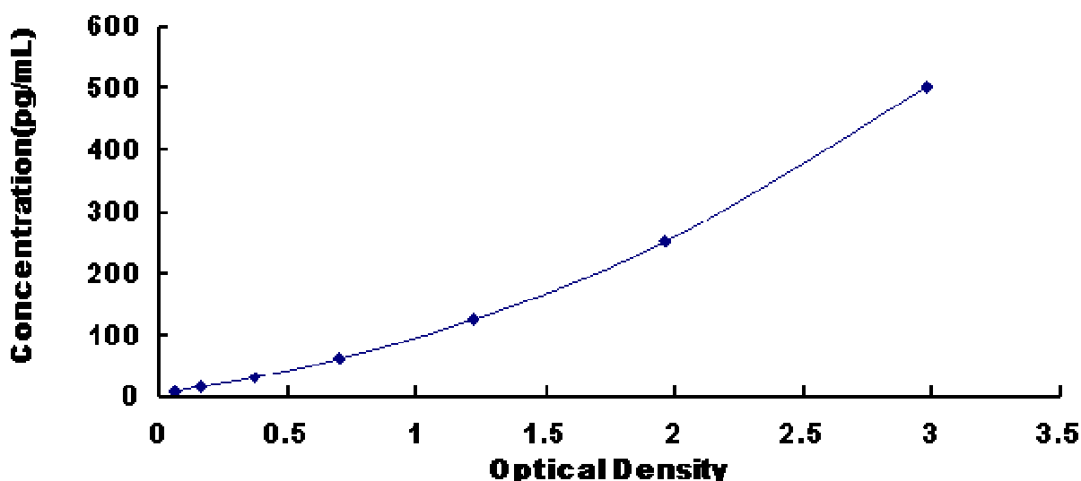
犬 N 端前脑钠素(NT-ProBNP)试剂盒标准曲线
