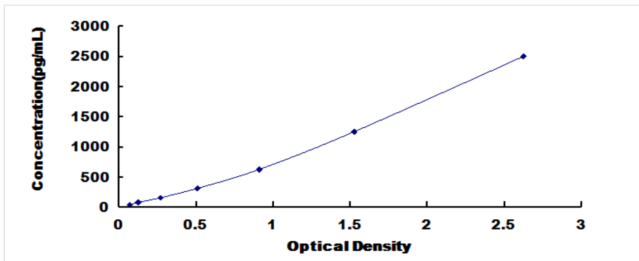
人氨基端前脑钠素 (NT-ProBNP) 检测试剂盒标准曲线
