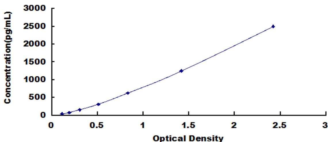
人氨基端前脑钠素 (NT-ProBNP) 检测试剂盒标准曲线
