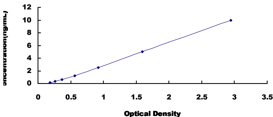
人 NADH 脱氢酶 5 (ND5) 试剂盒标准曲线
