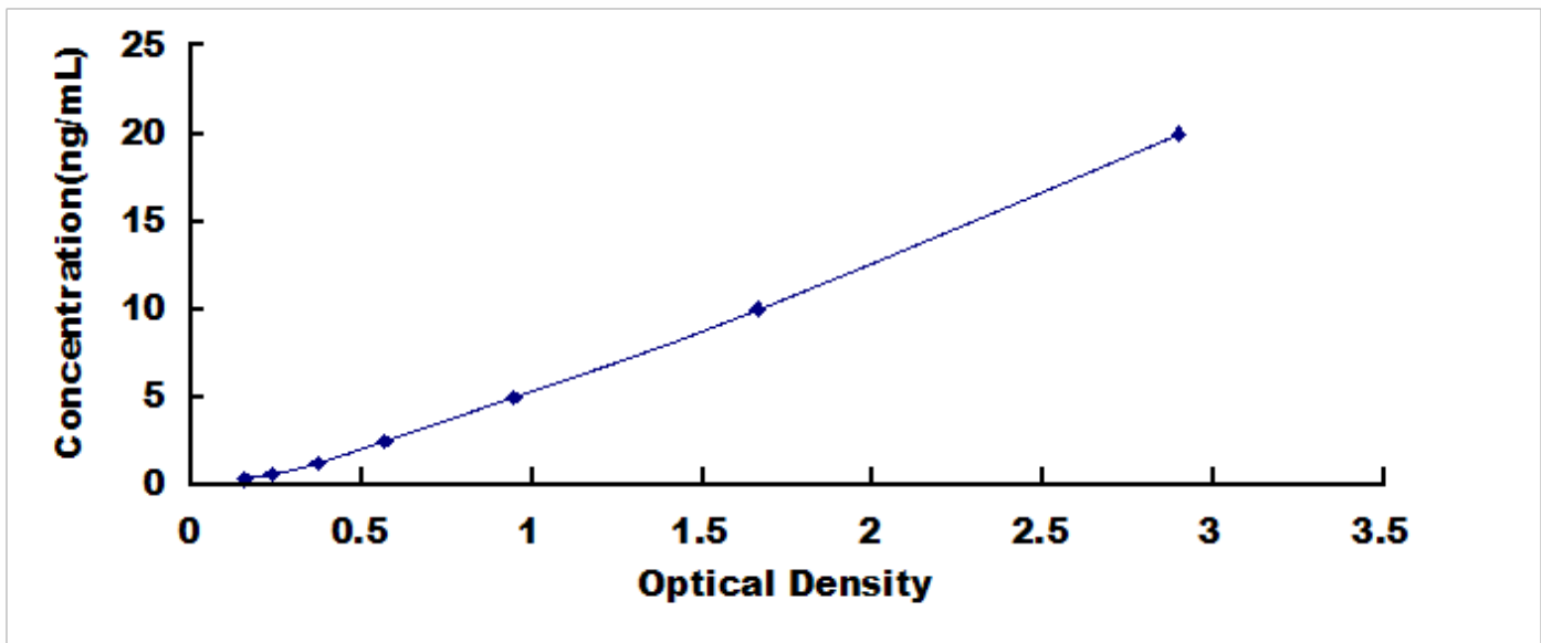
人 NEDD4 结合蛋白 2 (N4BP2) 检测试剂盒标准曲线
