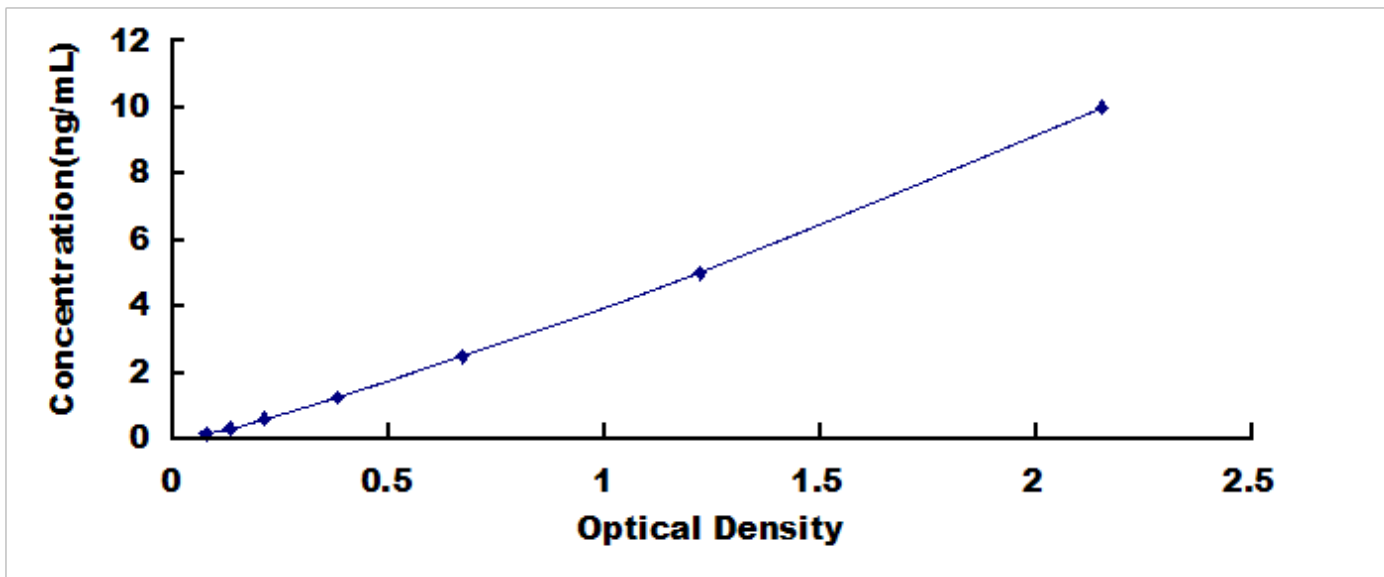
人 NFkB 激活蛋白 (NKAP) 检测试剂盒标准曲线
