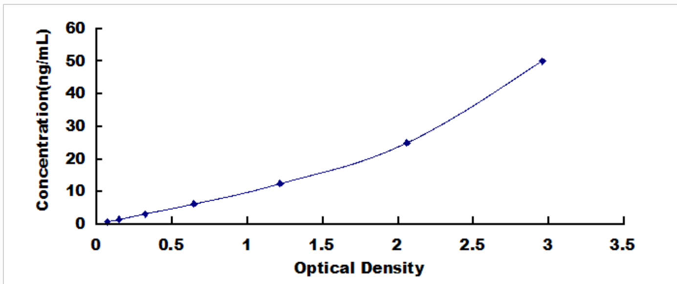
人 Na + 牛磺胆共转运多肽 (NTCP) 检测试剂盒标准曲线
