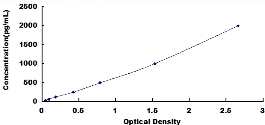
兔神经生长因子(NGF)检测试剂盒标准曲线
