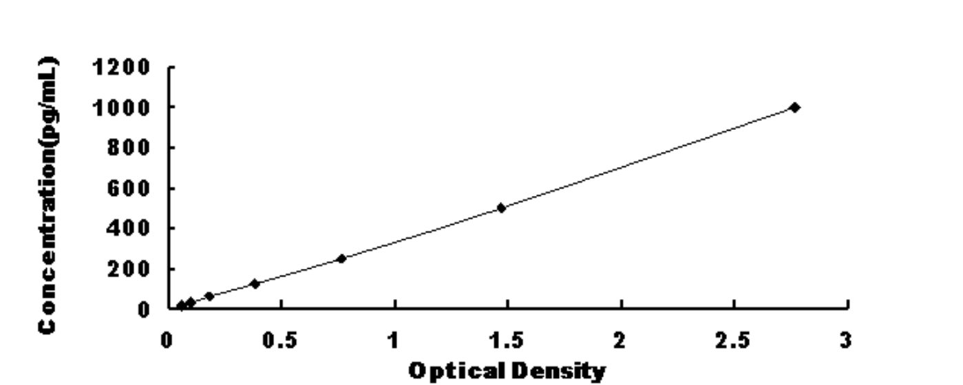
大鼠脑红蛋白(NGB)试剂盒标准曲线
