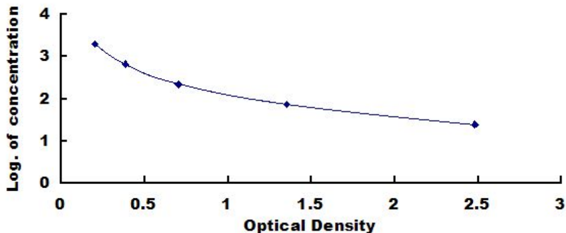
人神经肽 Y (NPY) 检测试剂盒标准曲线
