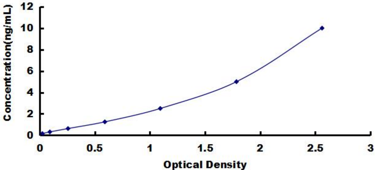
人中性鞘磷脂酶 (NSMASE) 检测试剂盒标准曲线
