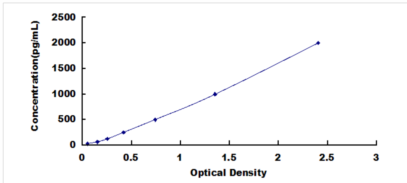
人中性粒细胞明胶酶关联脂质运载蛋白 (NGAL) 检测试剂盒标准曲线
