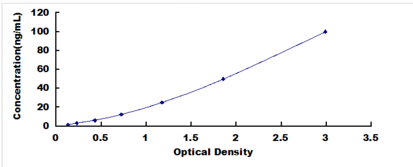
犬中性粒细胞明胶酶关联脂质运载蛋白 (NGAL) 检测试剂盒标准曲线
