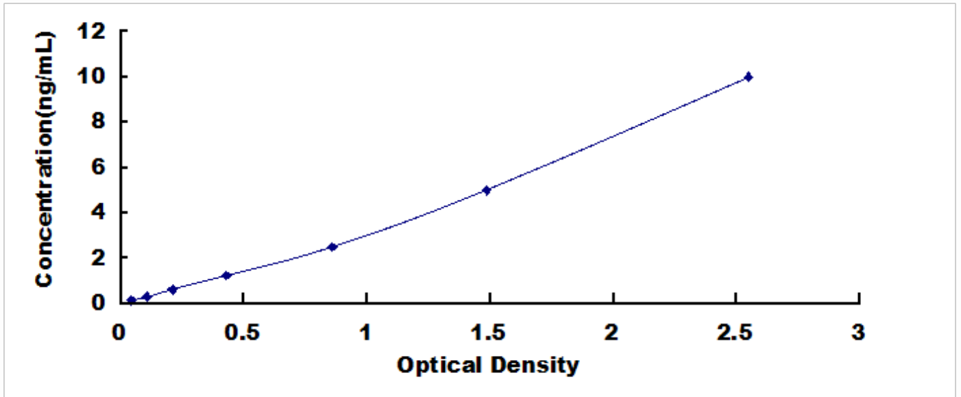
人尼克酰胺腺嘌呤二核苷酸磷酸氧化酶 4 (NOX4) 检测试剂盒标准曲线
