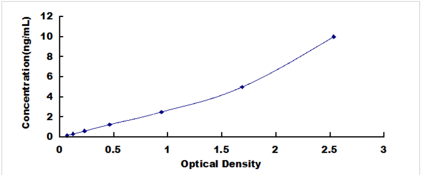
人核因子 \kappa B (NF \kappa B) 检测试剂盒标准曲线
