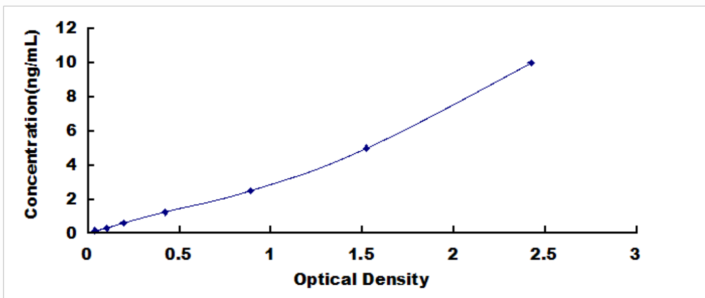
人 O-6-甲基鸟嘌呤 DNA 甲基转移酶 (MGMT) 检测试剂盒标准曲线
