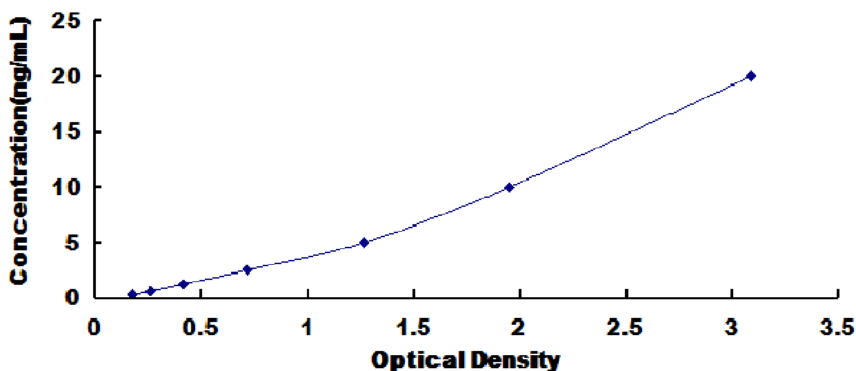
人有机溶质载体伴侣 1(OSCP1)检测试剂盒标准曲线
