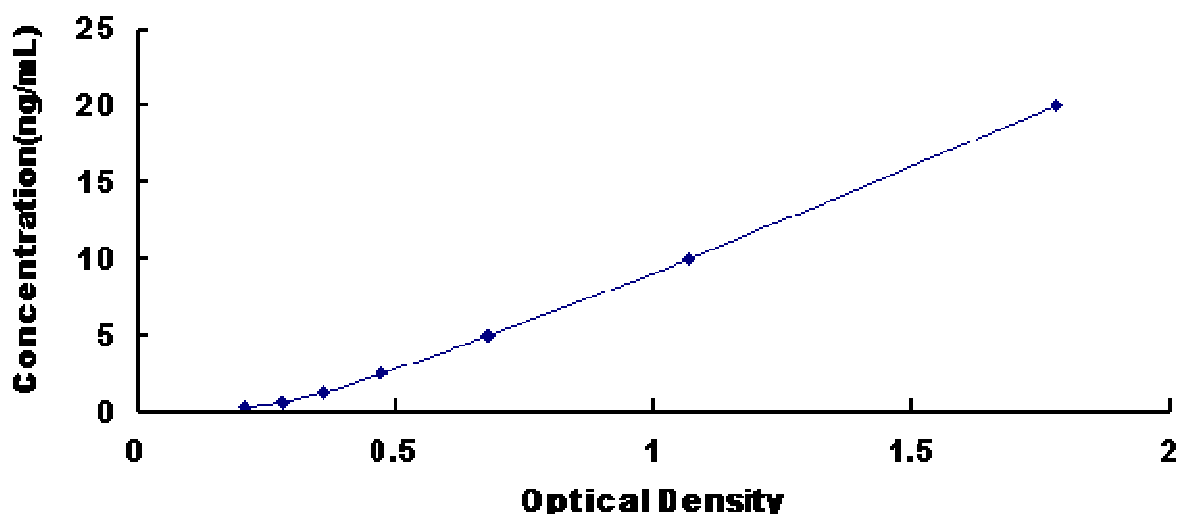
人骨粘连蛋白(ON)试剂盒标准曲线
