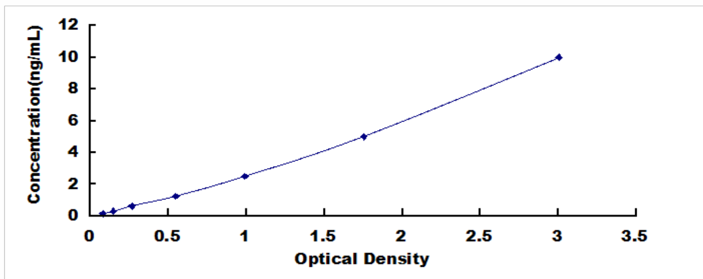
小鼠骨保护素(OPG)检测试剂盒标准曲线
